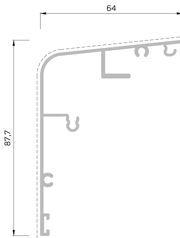
BBC1496 ghidaj inferior 0.622 kg/ml
