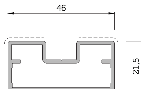
BBC1496 ghidaj inferior 0.622 kg/ml
