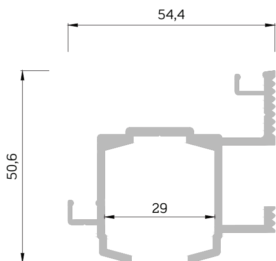
BBC4390 ghidaj superior 0.992 kg/ml
